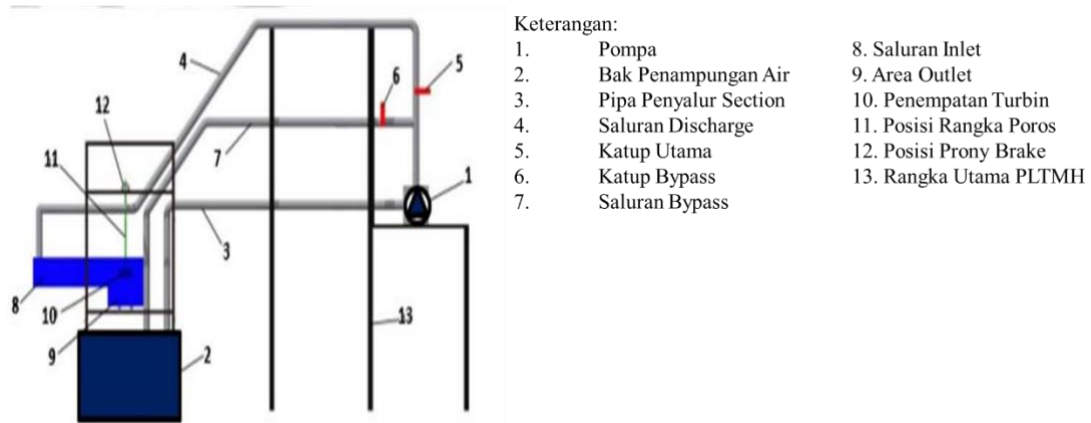
Gambar 1 Setup eksperimen
