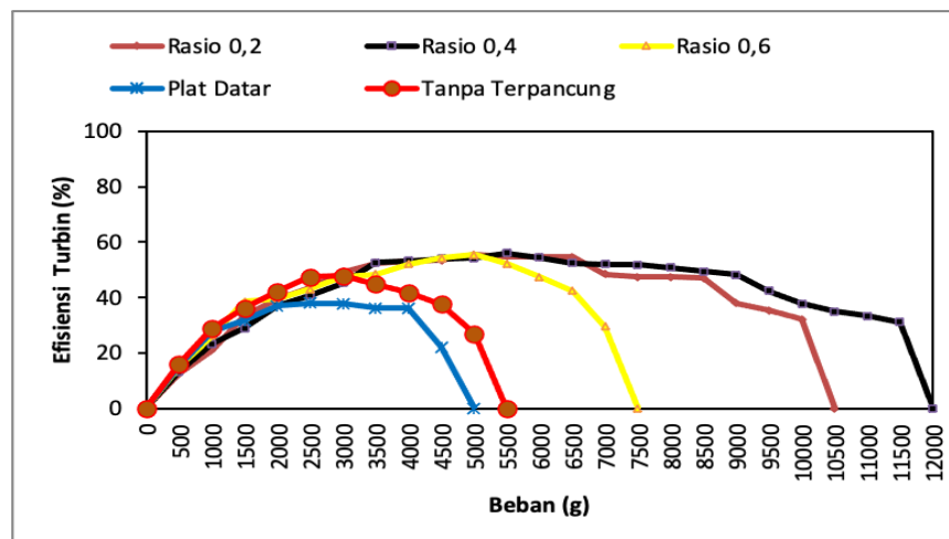
Gambar 7 Efisiensi turbin pada kapasitas 14,322 L/s
