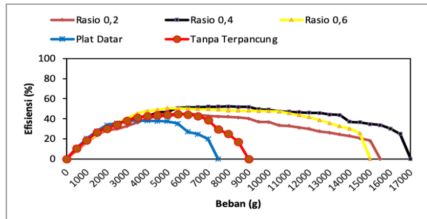
Gambar 8 Efisiensi turbin pada kapasitas 18,113 L/s
