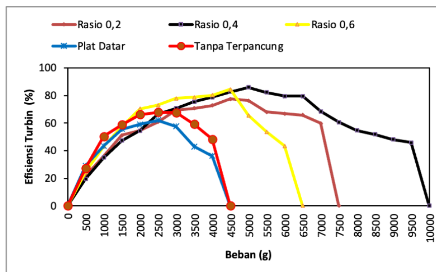
Gambar 6 Efisiensi turbin pada kapasitas 11,024 L/s
